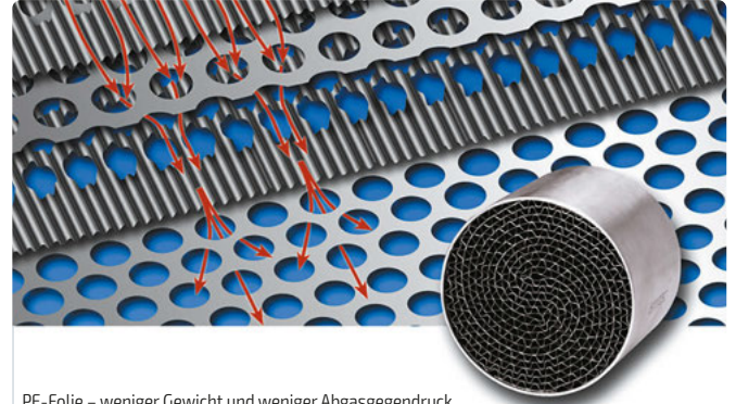
PE-Folie – weniger Gewicht und weniger Abgasgegendruck
